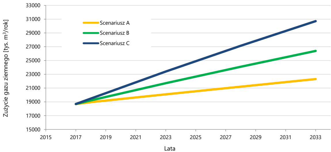
Wykres 4.2 Prognozowane zmiany zużycia gazu ziemnego do roku 2033
