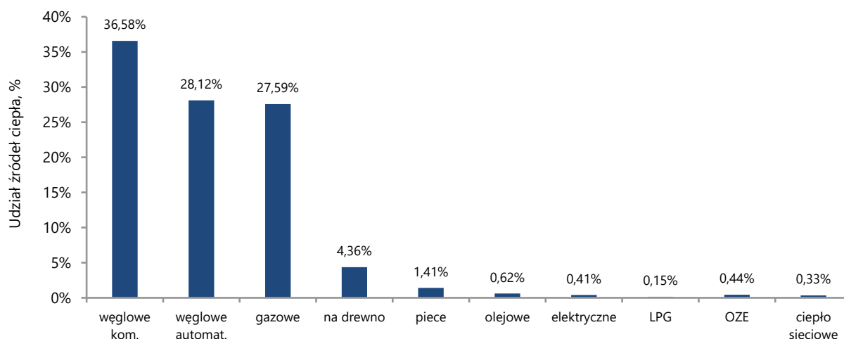
Wykres 3.9 Struktura źródeł ciepła w budownictwie indywidualnym do celów grzewczych
